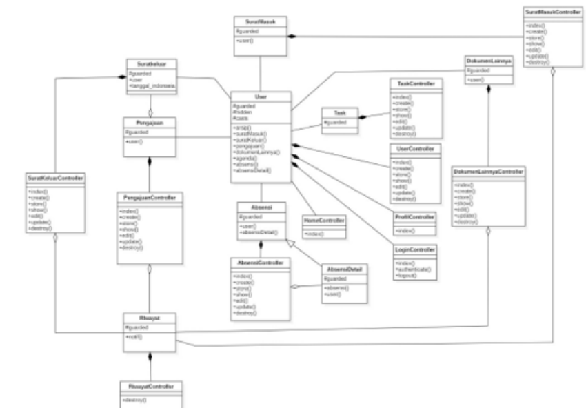
Gambar 3. 41 Class Diagram Sistem Informasi Manajemen Administrasi
