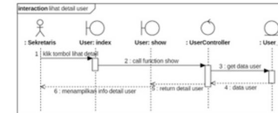
Gambar 3. 23 Sequence Diagram Lihat Detail Pengguna
