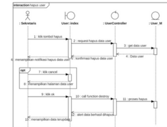
Gambar 3. 24 Sequence Diagram Hapus Pengguna
